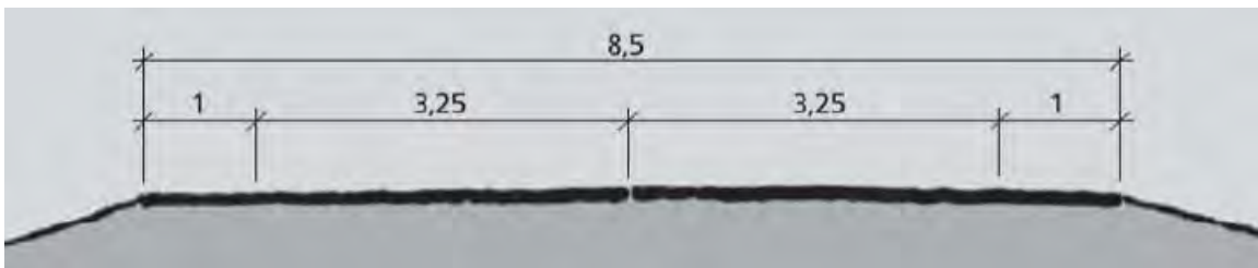
Fig 3-14. Vegprofil – ny E6 Sørrelva – Borkamo.
